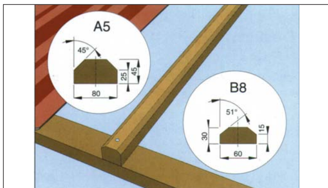
Montáž svislé podkladní latě
