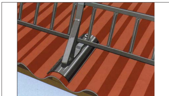
Příložka univerzální v kombinaci s mříží sněholamu
